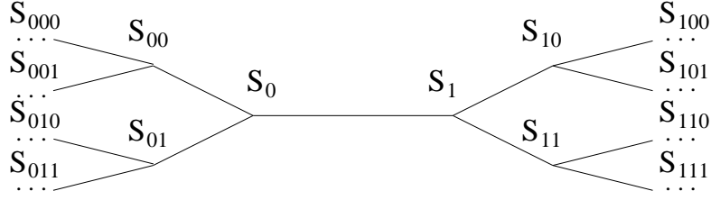
FIG. 2: Arbre de \mathbb{C}_2 - \mathcal{O}_{\mathbb{Q}_2} .
