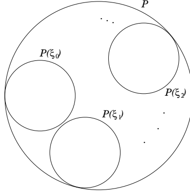
FIG. 4: Chaque bout \mathcal{P} d'une composante analytique de \mathcal{E}(R) a une infinité de disques de Siegel attachés.
