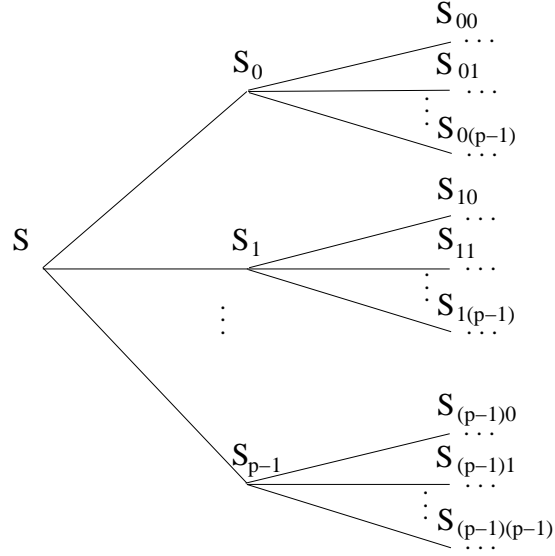
FIG. 1: Arbre de \mathbb{C}_p - \mathcal{O}_{\mathbb{Q}_p} , pour p > 2 .
