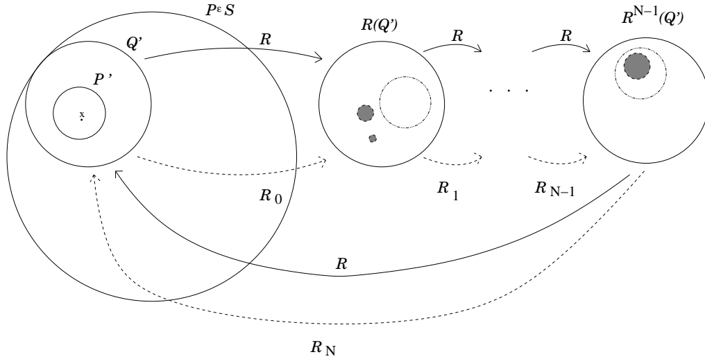
FIG. 3: La partie noire représente le complémentaire de I .
